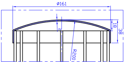
Detail:X SCALE 2:1
