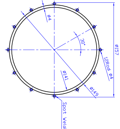
SEC:B-B SCALE 2:1
