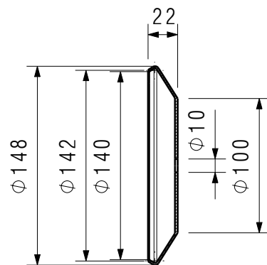
POS 2 BOTTOM CAP
