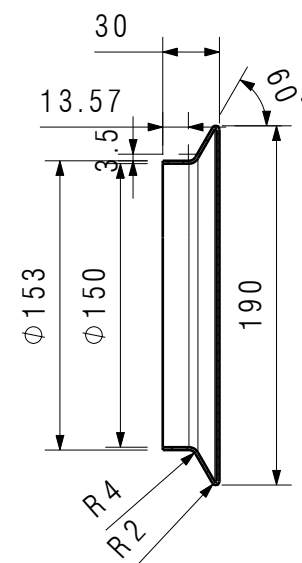
POS 3 TOP CAP
