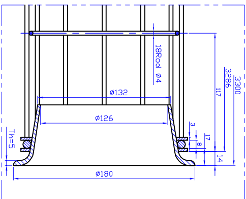
Detail:Z SCALE 2:1
