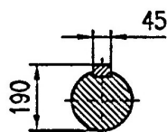
Schnitt A-B Section A-B
